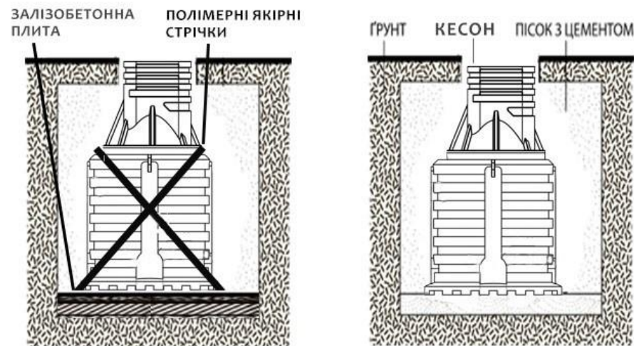
Рис.2 – Схематичне зображення монтажу ємності
